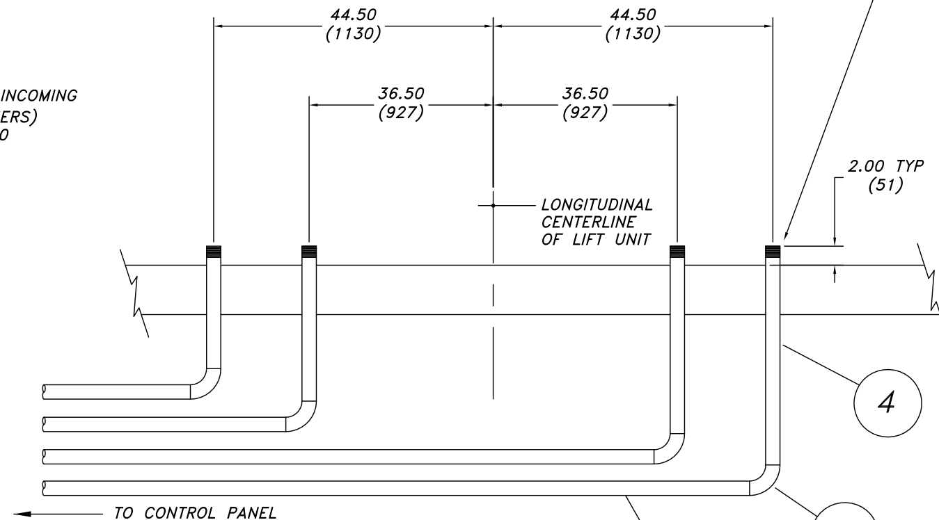
SECTION D-D
